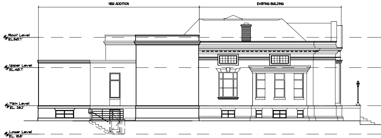
2 EAST ELEVATION A-6 SCALE: 1/16" = 1'-0"
